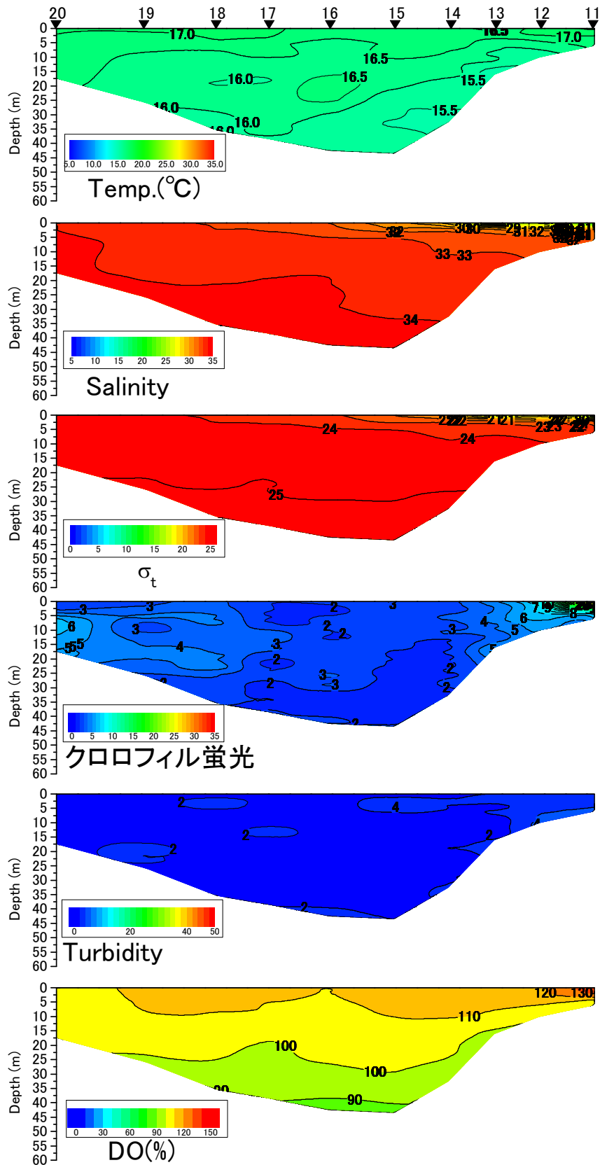
八代海中央ラインの水温(°C)、塩分、密度( \sigma_t )、クロロフィル蛍光強度、濁度、溶存酸素飽和度(DO%)の鉛直面図(国土交通省の調査による) (2017年4月21日)
